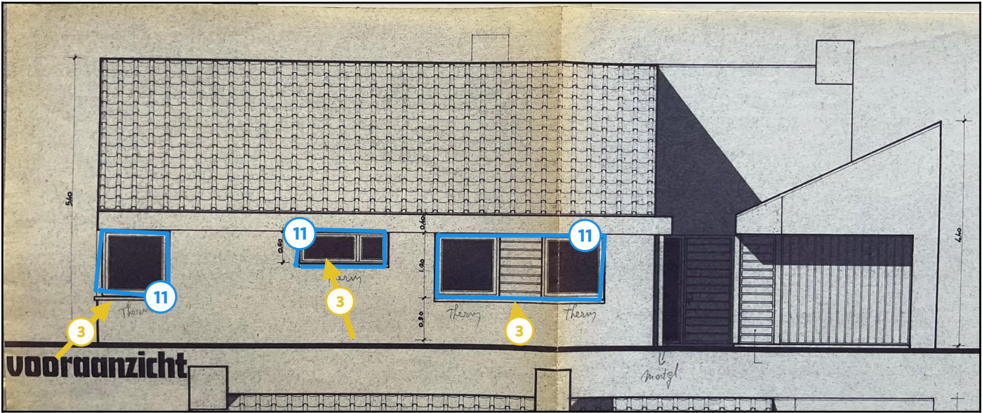
Legende van plan 1.7: Voorgevel
