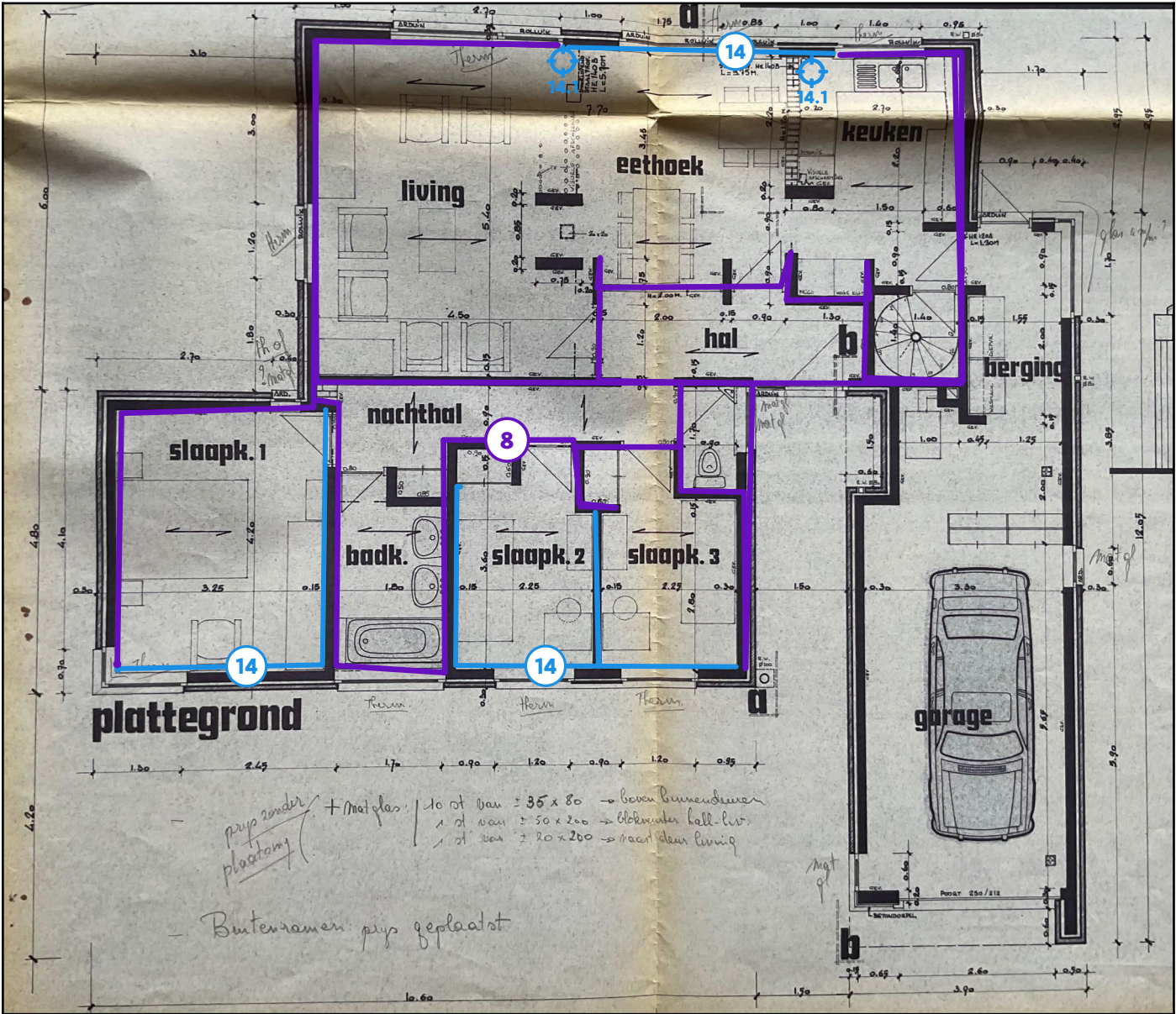
Legende van plan 1.3: Gelijkvloers wanden
